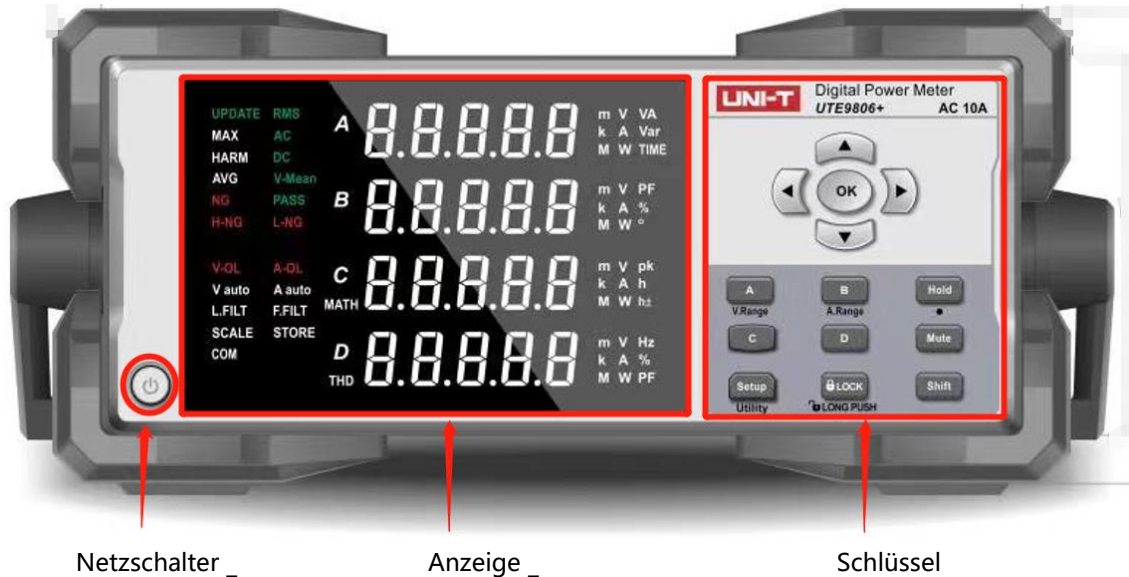
Abbildung 2.3. 2 UTE9806+ Frontplatte
