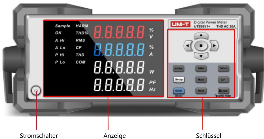
Abbildung 2.3. 3 UTE9811+ Frontplatte
